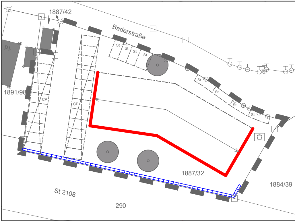
Abbildung 1: Lageplan mit Kennzeichnung der Lage der Lärmschutzwand und Kennzeichnung der Bereiche und der Fassaden, an denen Schallschutzmaßnahmen erforderlich sind
