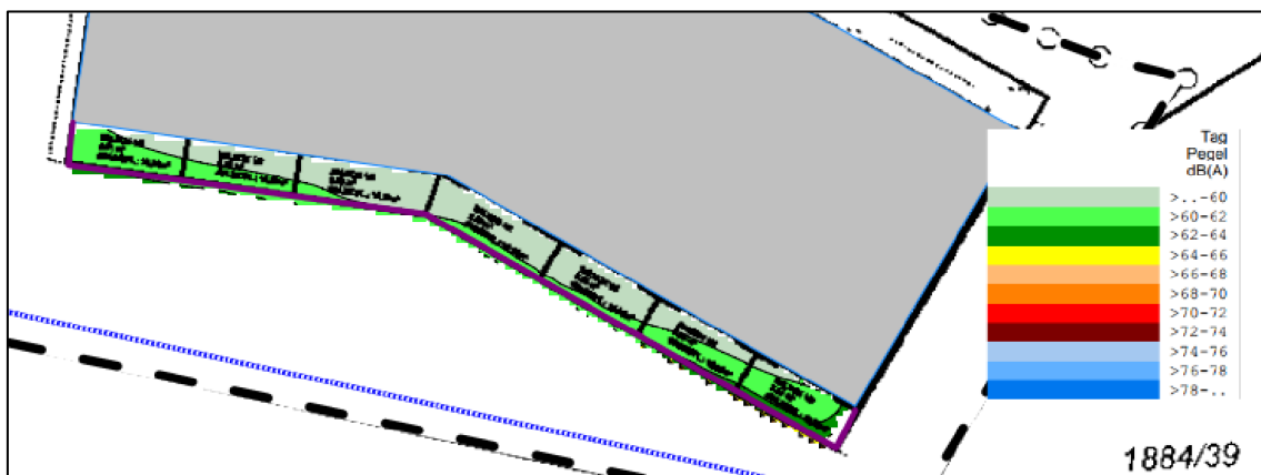
Abbildung 4: Exemplarische Darstellung der Geräuschkarte auf den südlichen Balkonen des zweiten Obergeschosses (Brüstungshöhe von h = 1,20 \text{ m} über FOK)
